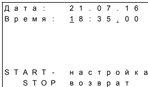
Рис.25. Установка даты и времени
