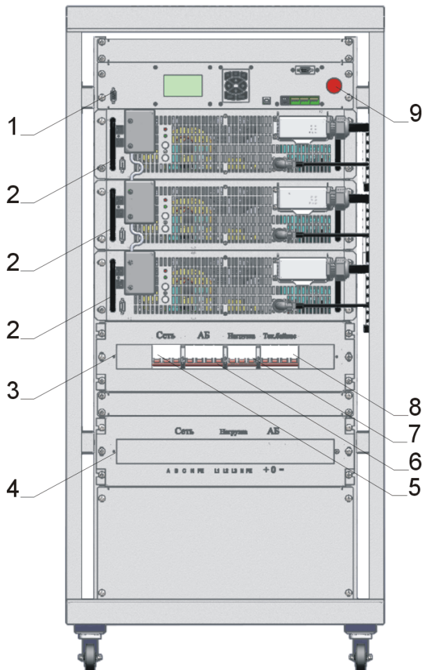
Рис. 1 ИБП РПД-3/3-30-380. Вид спереди.
