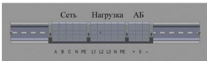
Рис.4 Клеммные колодки ИБП
