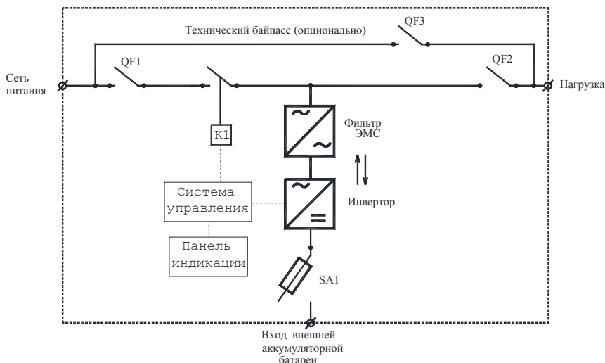
Рис. 3 Структурная схема ИБП
